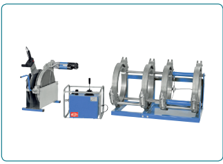
WIDOS 4911
