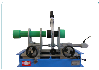
WIDOS 35XX
