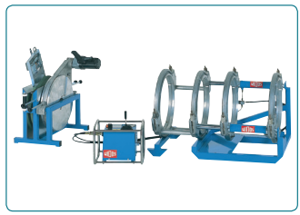
WIDOS 5100 - 6100
