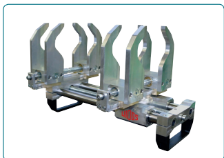
WIDOS JIG
