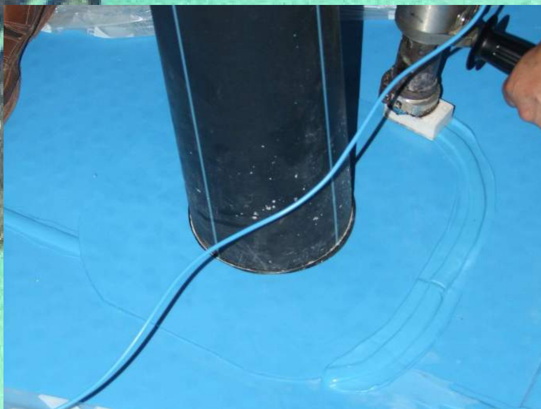
DE Detailansicht Rohrdurchführungsmontage // CZ Detail montáže průchodu roury
